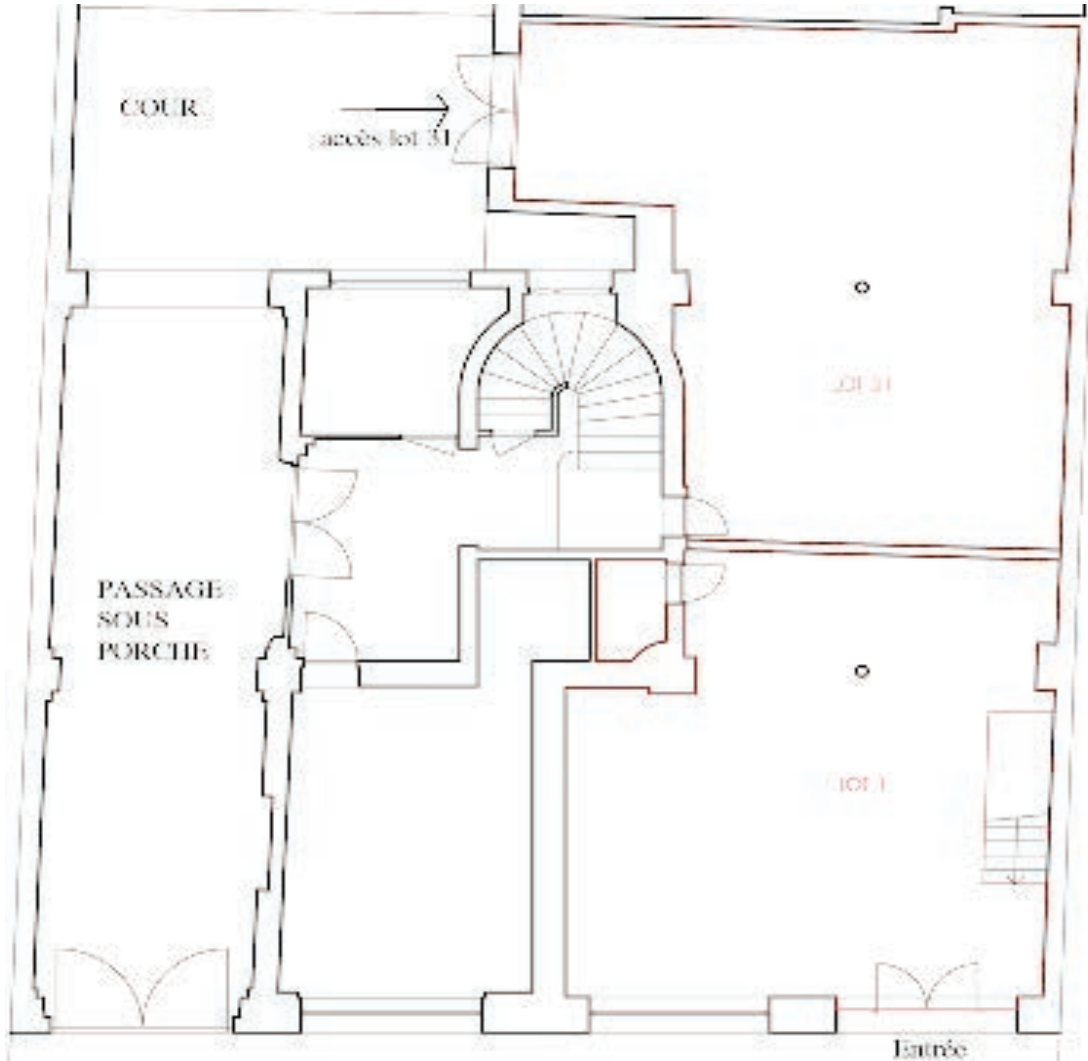
Plan du rez-de-chaussée, sans valeur contractuelle
